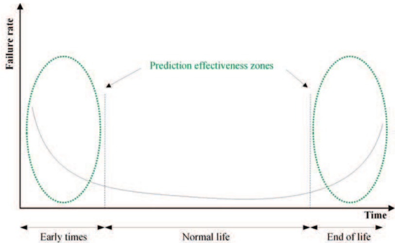
Fig. 1 - Valutazione delle zone di efficacia di previsione: tasso di malfunzionamento funzione della vita utile.
